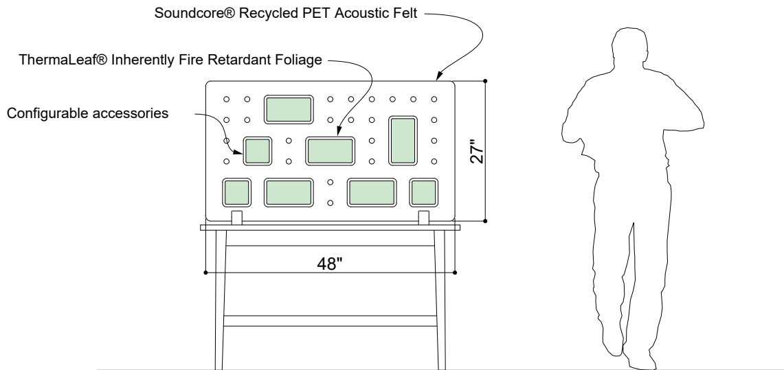
② ELEVATION 2
