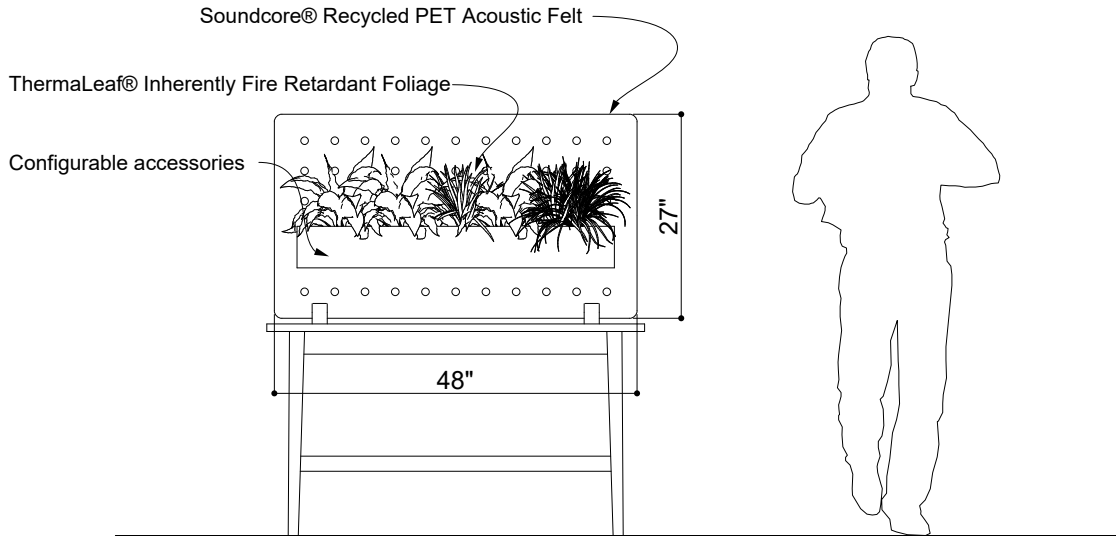
① ELEVATION 1
